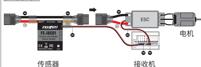
接线方式二：
