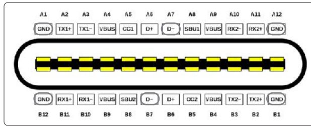
Type-C 接口图
