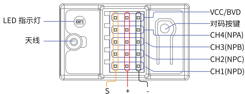
FGr4B 接收机概览图
