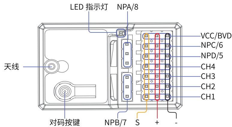
FGr8B 接收机概览图
