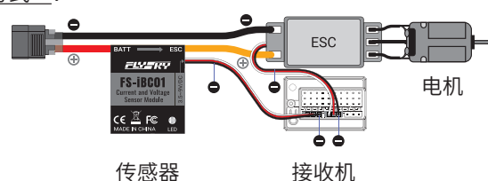
接线方式一：
